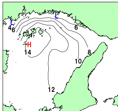
透明度（m）
