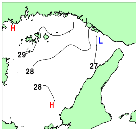
水温（表層、℃）
