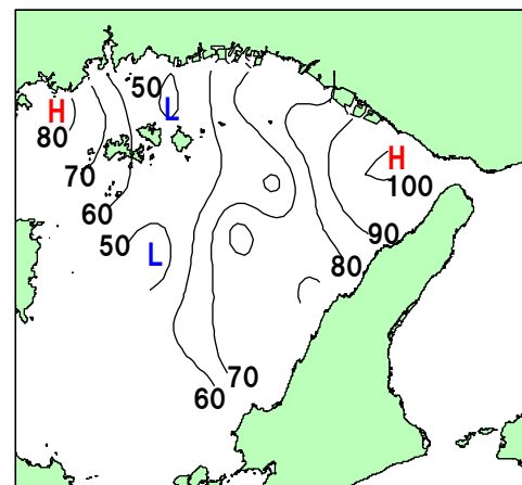
溶存酸素量（底層、%）
