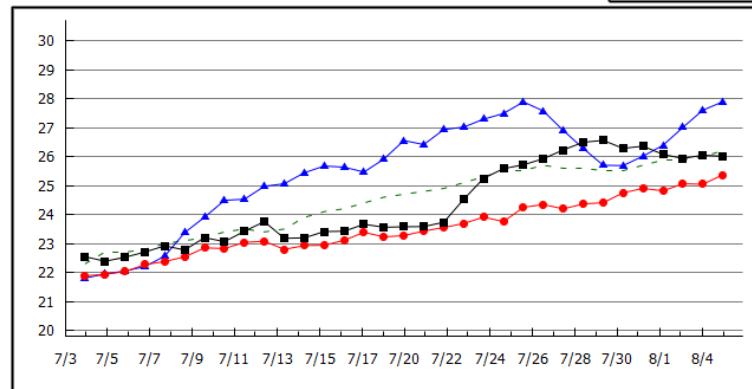
2019年08月05日 坊勢(水温) 表層: 26.0℃ 昨年表層: 27.9℃ 底層: 25.4℃ 今年表層: 26.0℃ 昨年表層: 27.9℃ 底層: 25.4℃ 今年底層: 25.4℃ 今年表層: 26.0℃ 昨年表層: 27.9℃
