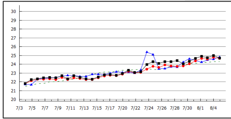
2019年08月05日 交流の翼港(水温) 表層: 24.7℃ 昨年表層: 24.8℃ 底層: 24.7℃ 今年表層: 24.7℃ 昨年表層: 24.8℃ 底層: 24.7℃ 今年底層: 24.7℃ 今年表層: 24.7℃
