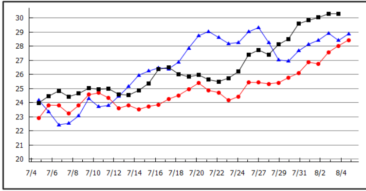
2019年08月05日 室津(水温) 表層: 30.6℃ 昨年表層: 28.9℃ 底層: 28.4℃ 今年表層: 30.6℃ 昨年表層: 28.9℃ 底層: 28.4℃ 今年底層: 28.4℃ 今年表層: 30.6℃
