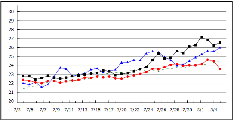
2019年08月05日 沼島(水温) 表層: 26.5℃ 昨年表層: 26.0℃ 底層: 23.6℃ 今年表層: 26.5℃ 昨年表層: 26.0℃ 底層: 23.6℃ 今年底層: 23.6℃ 今年表層: 26.5℃ 昨年表層: 26.0℃
