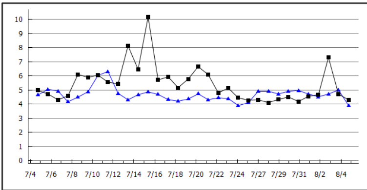
2019年08月05日:4.3 室津(加齢) 昨年: 3.9 今年: 4.3 今年表層: 4.3 昨年表層: 3.9 今年底層: 4.3 昨年底層: 3.9 今年表層: 4.3 昨年表層: 3.9
