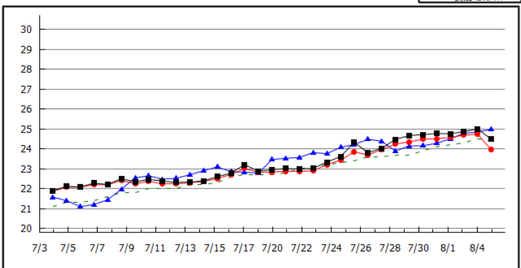
2019年08月05日 福良(水温) 表層: 24.5℃ 昨年表層: 25.0℃ 底層: 24.0℃ 今年表層: 24.5℃ 昨年表層: 25.0℃ 底層: 24.0℃ 今年底層: 24.0℃ 今年表層: 24.5℃ 昨年表層: 25.0℃
