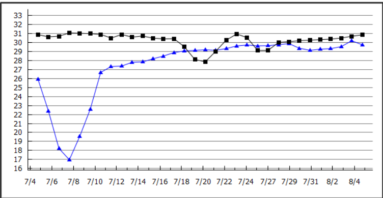
2019年08月05日:30.9 室津(塩分) 昨年: 29.8 今年: 30.9 今年表層: 30.9 昨年表層: 29.8 今年底層: 30.9 昨年底層: 29.8 今年表層: 30.9 昨年表層: 29.8
