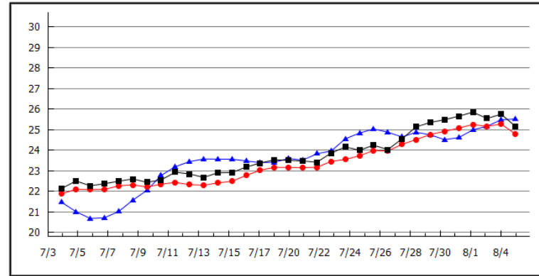
2019年08月05日 丸山(水温) 表層: 25.2℃ 昨年表層: 25.5℃ 底層: 24.8℃ 今年表層: 25.2℃ 昨年表層: 25.5℃ 底層: 24.8℃ 今年底層: 24.8℃ 今年表層: 25.2℃ 昨年表層: 25.5℃
