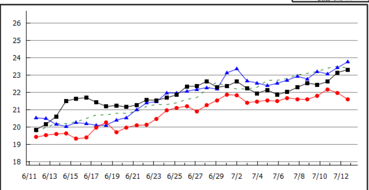
2020年07月13日 坊勢(水温) 表層: 23.3℃ 昨年表層: 23.8℃ 底層: 21.6℃ 平年値: 23.4℃
