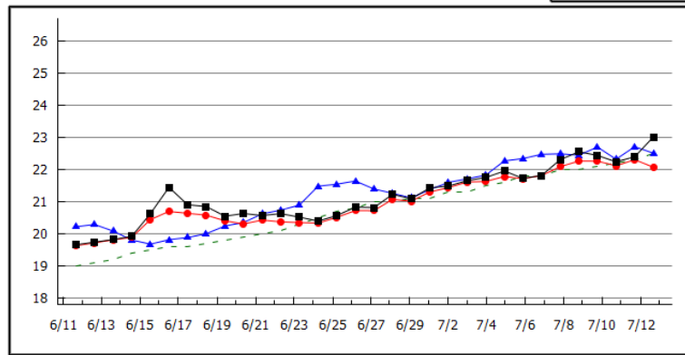
2020年07月13日 交流の翼港(水温) 表層: 23.0℃ 昨年表層: 22.5℃ 底層: 22.1℃ 平年値: 22.5℃
