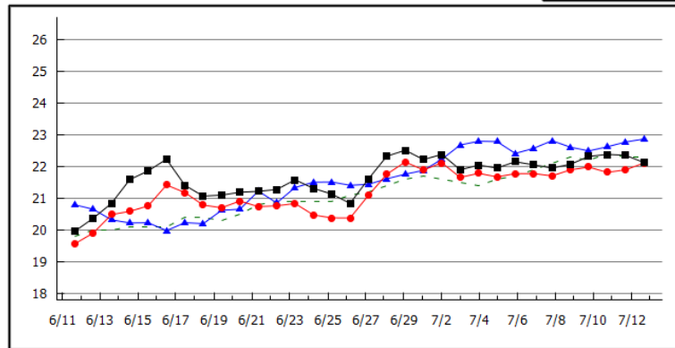
2020年07月13日 福良(水温) 表層: 21.9℃ 昨年表層: 22.3℃ 底層: 21.8℃ 平年値: 22.0℃
