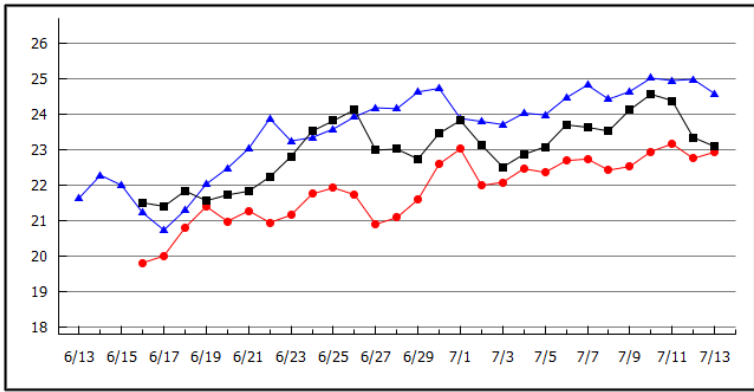
2020年07月13日 室津(水温) 表層: 23.1℃ 昨年表層: 24.6℃ 底層: 22.9℃ 平年値: ---℃
