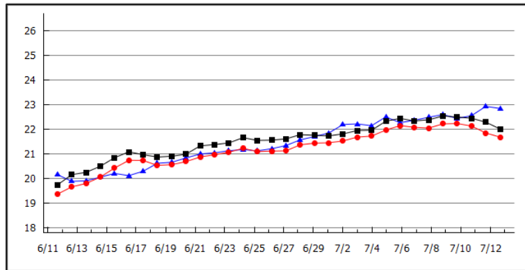
2020年07月13日 丸山(水温) 表層: 22.0℃ 昨年表層: 22.8℃ 底層: 21.7℃ 平年値: ---℃
