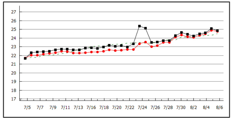
交流の翼港(水温) 2018年08月06日 表層 : 24.8 °C 昨年表層 : --- °C 底層 : 24.8 °C 平年値 : 24.5 °C
