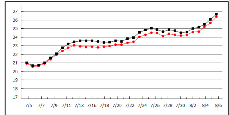
丸山(水温) 2018年08月06日 表層 : 26.7 °C 昨年表層 : --- °C 底層 : 26.4 °C 平年値 : --- °C
