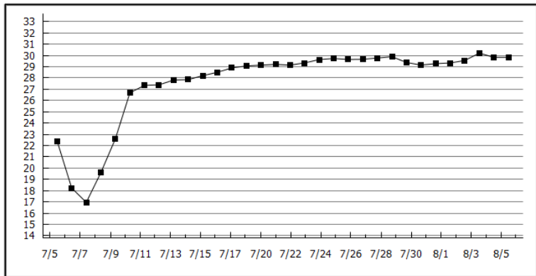
室津(塩分) 2018年08月06日:29.8 昨年 : --- 平年値 : ---
