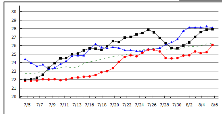
坊勢(水温) 2018年08月06日 表層 : 27.9 °C 昨年表層 : 28.1 °C 底層 : 26.1 °C 平年値 : 26.3 °C
