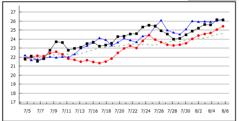
沼島(水温) 2018年08月06日 表層 : 26.1 °C 昨年表層 : 26.2 °C 底層 : 25.4 °C 平年値 : 24.6 °C
