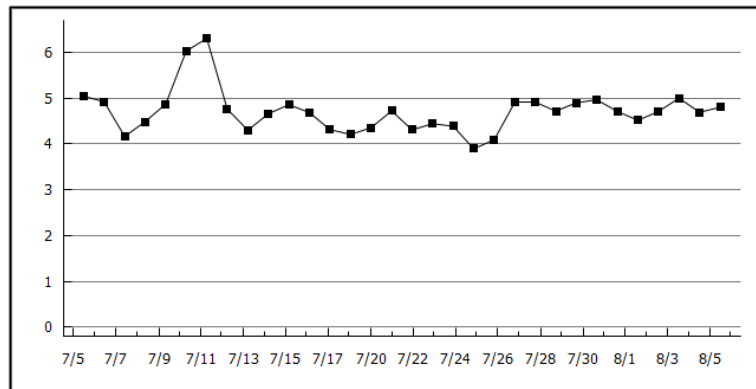
室津(加齢7代) 2018年08月06日:4.8 昨年 : --- 平年値 : ---
