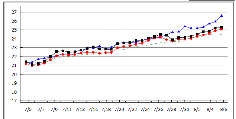
福良(水温) 2018年08月06日 表層 : 25.3 °C 昨年表層 : 26.6 °C 底層 : 25.1 °C 平年値 : 24.5 °C
