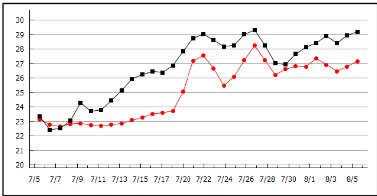
室津(水温) 2018年08月06日 表層 : 29.2 °C 昨年表層 : --- °C 底層 : 27.2 °C 平年値 : --- °C
