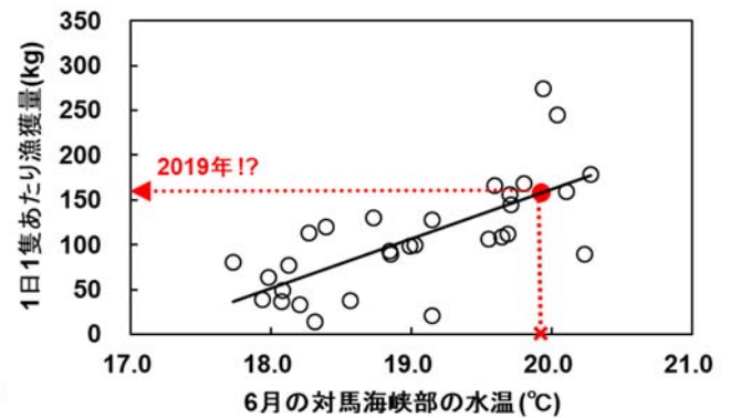
図1：6月の水温と漁期中の来遊量指標値との関係
