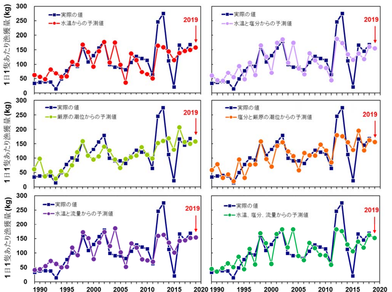
図2：対馬海峡部の6月の環境条件から予測した9～11月の来遊量指標値
