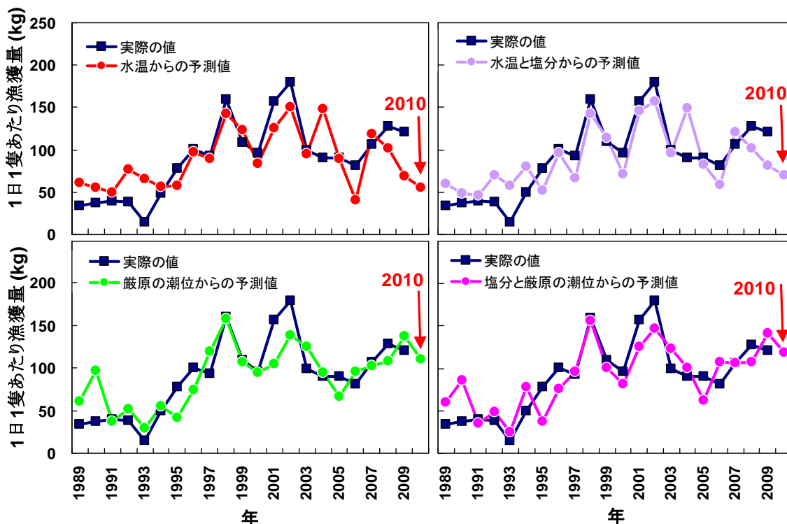
図2：6月の環境条件から予測した9～11月の来遊資源水準
