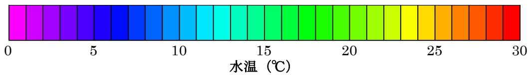
三尾沖（上図）、柴山沖（中央図）及び津居山沖（下図）の水深120m以浅の水温断面図
