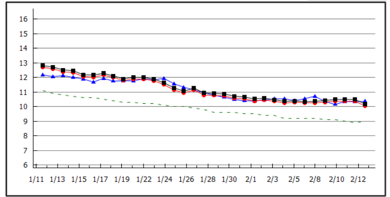
2024年02月13日 交流の翼港(水温) 表層: 10.2 °C 昨年表層: 10.4 °C 底層: 10.0 °C 平年値: 9.0 °C
