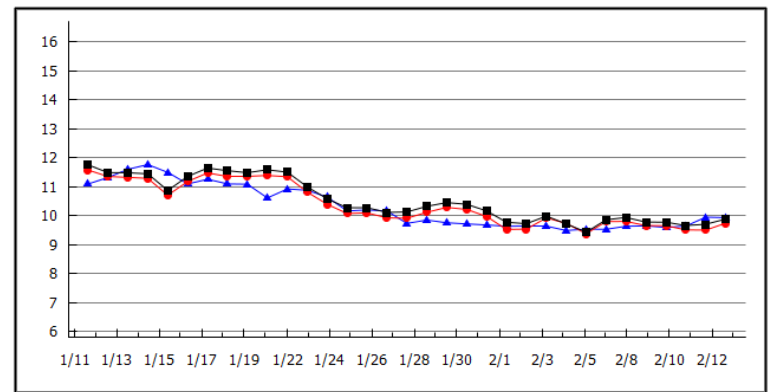
2024年02月13日 丸山(水温) 表層: 9.9 °C 昨年表層: 9.9 °C 底層: 9.7 °C 平年値: --- °C
