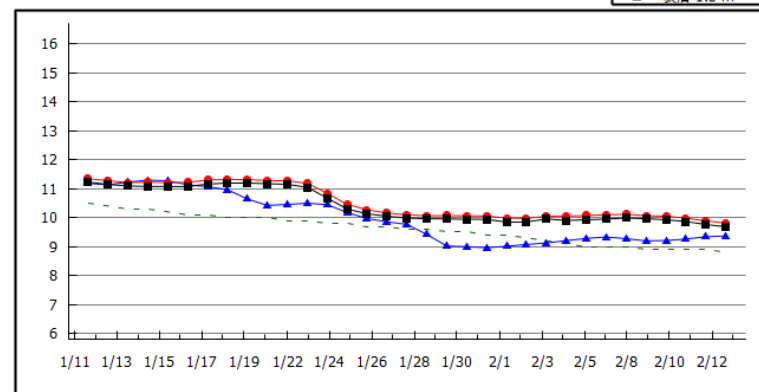
2024年02月13日 坊勢(水温) 表層: 9.7 °C 昨年表層: 9.4 °C 底層: 9.8 °C 平年値: 8.8 °C
