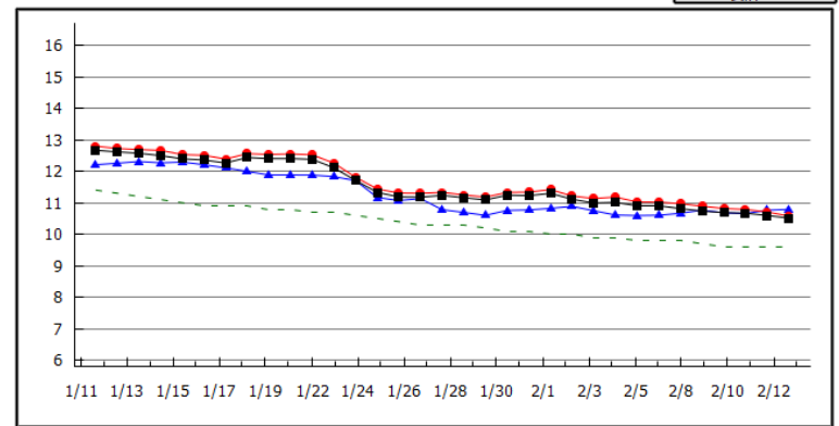
2024年02月13日 福良(水温) 表層: 10.5 °C 昨年表層: 10.8 °C 底層: 10.6 °C 平年値: 9.6 °C
