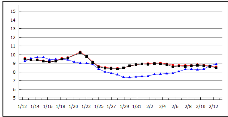
2024年02月13日 室津(水温) 表層: 8.5 °C 昨年表層: 8.9 °C 底層: 8.6 °C 平年値: --- °C
