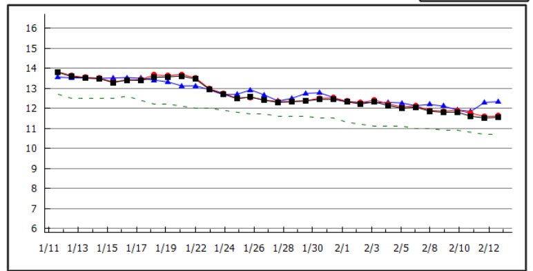
2024年02月13日 沼島(水温) 表層: 11.6 °C 昨年表層: 12.3 °C 底層: 11.6 °C 平年値: 10.7 °C
