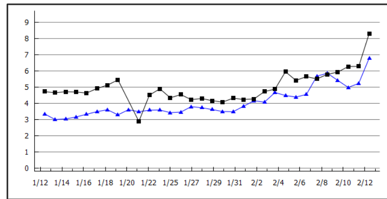
2024年02月13日:8.3 室津(加齢) 昨年: 6.8 平年値: ---
