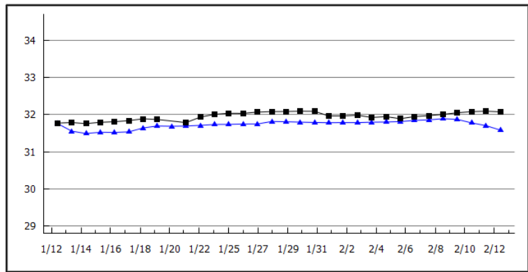
2024年02月13日:32.1 室津(塩分) 昨年: 31.6 平年値: ---
